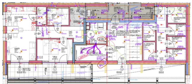
Übersicht Erdgeschoß
