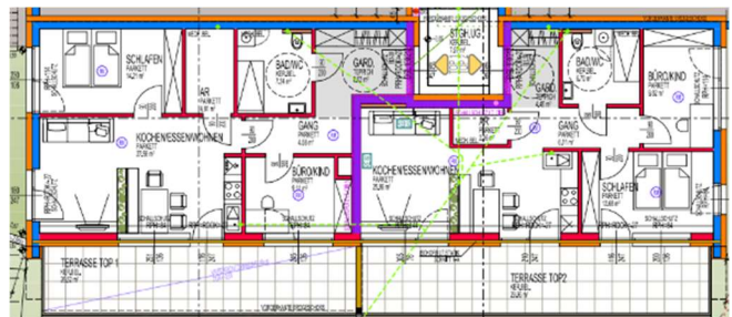
Übersicht Untergeschoß
