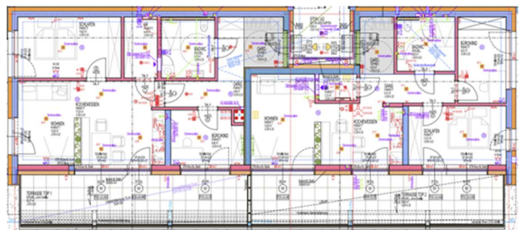
Übersicht Untergeschoß
